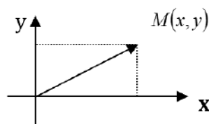
Figura2.3: Representación geométrica de número complejo.
