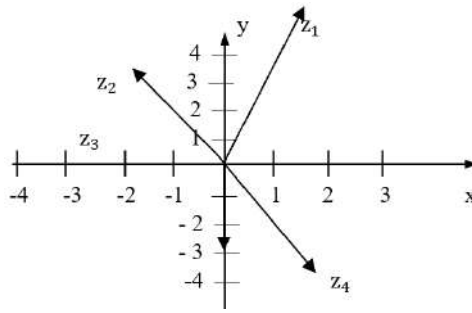
Figura 2.4: Geométrica de varios números complejos.
