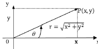
Figura 2.5: Forma polar de un número complejo.
