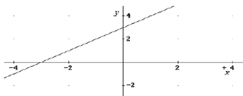
Figura 2.2: Representación gráfica función y = x + 3 .
